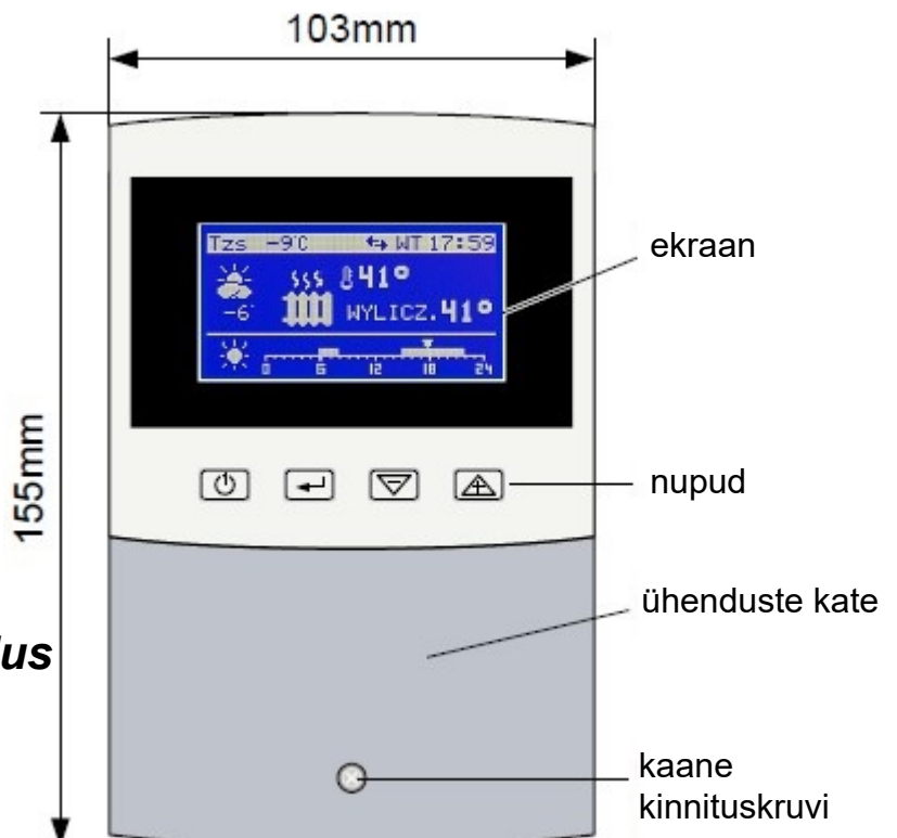
Joonis 11: BWC 310 regulaatori ehitus ja mõõtmed
