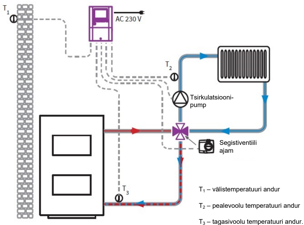
Joonis 3: Temperatuuri reguleerimine 4-suunalise ventiiliga.
