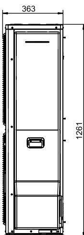
Außeneinheit BWL-1S(B)-10/14/16 Seitenansicht
