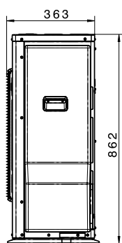
Außeneinheit BWL-1S(B)-05/07 Seitenansicht
