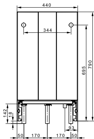
Inneneinheit Vorderansicht
