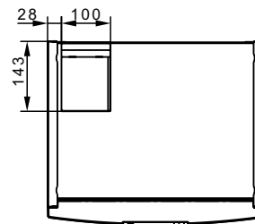
Inneneinheit Draufsicht
