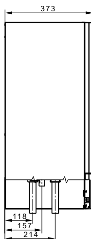
Inneneinheit Seitenansicht
